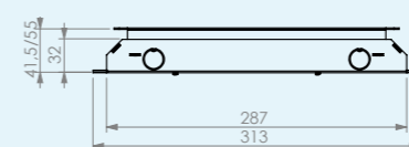
Dimensions combinées avec couvercle T15
