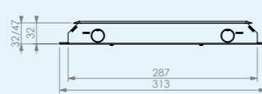
Dimensions combinées avec couvercle T3
